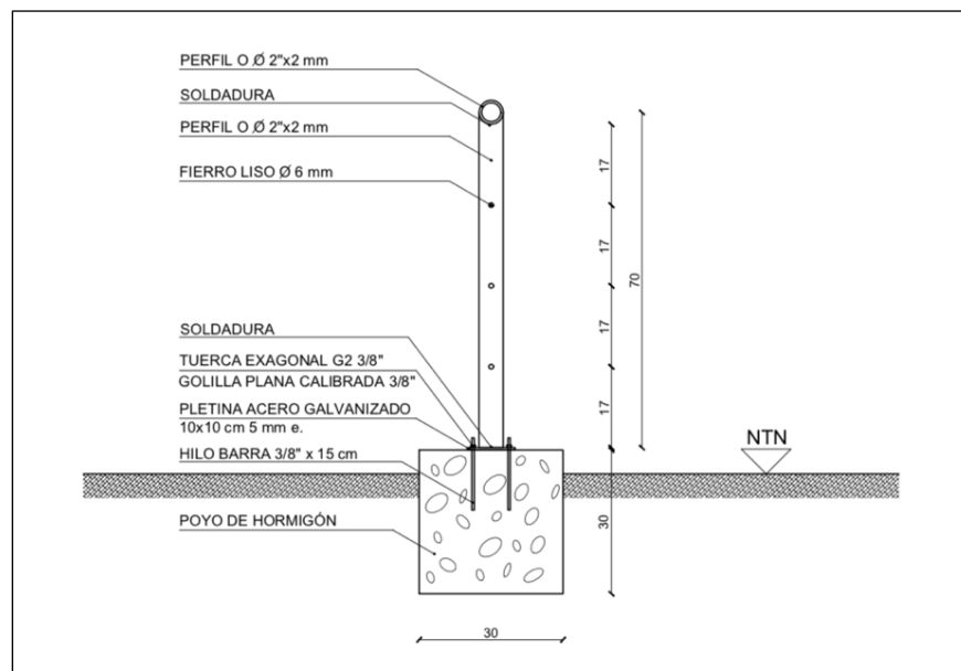
Imagen 16: Diseño propuesto cierres hallazgos
