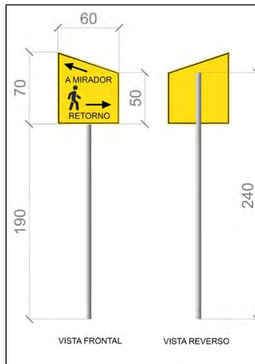
Imagen 10: Diseño propuesto señalética peatonal
