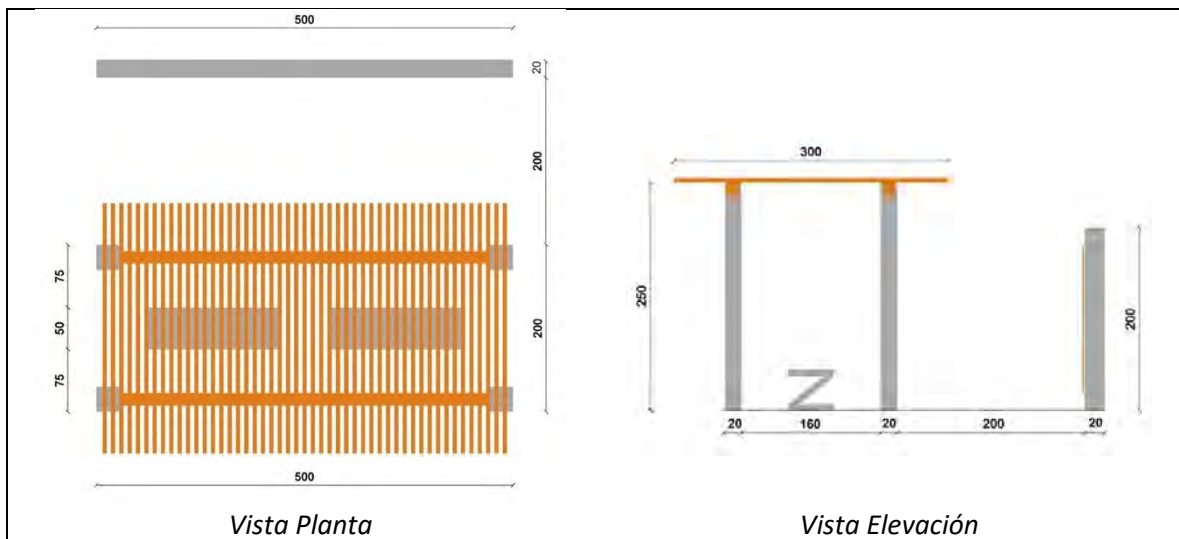
Imagen 8: Diseño propuesto sombreadero y dos bancas
