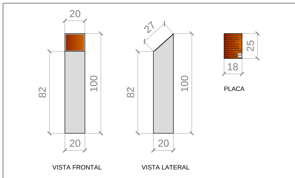
Imagen 9: Diseño propuesto pedestales con placas
