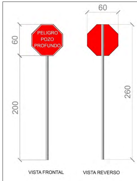
Imagen 13: Diseño propuesto señalética preventiva
