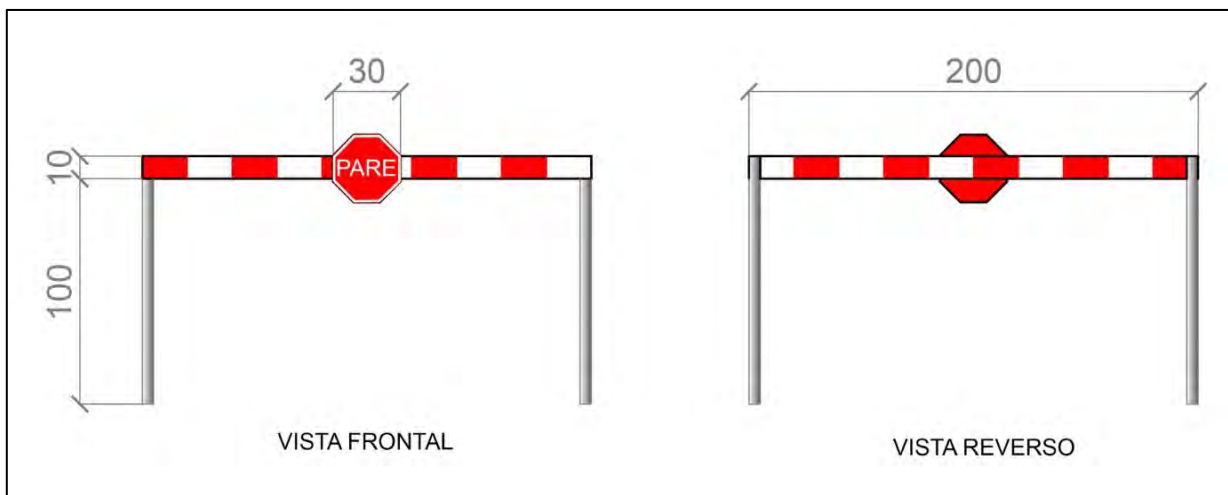
Imagen 3: Diseño propuesto Barreras
