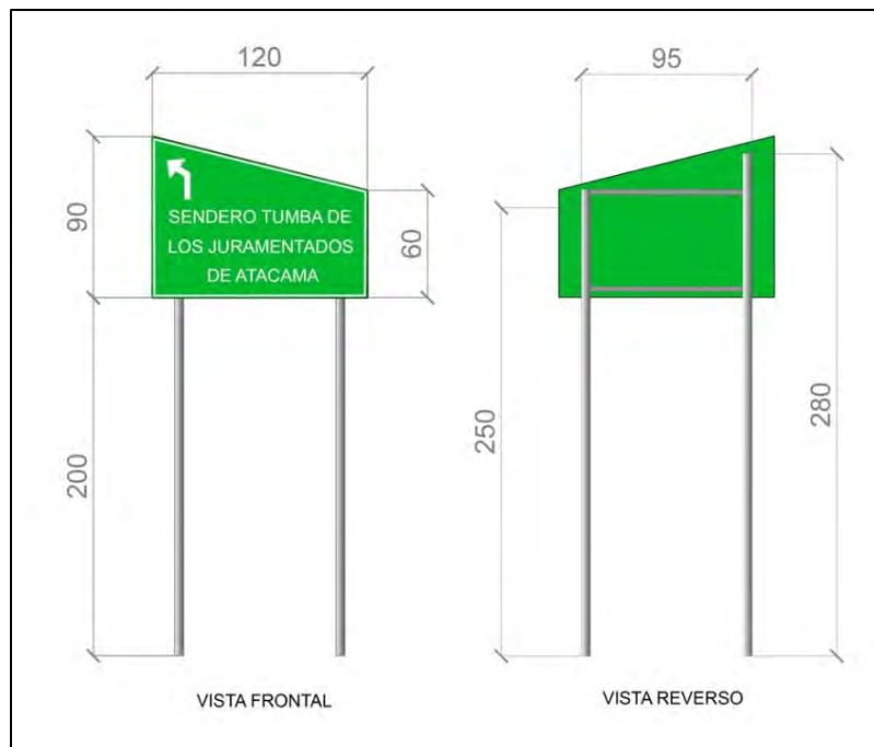
Imagen 4: Diseño propuesto señalética vial
