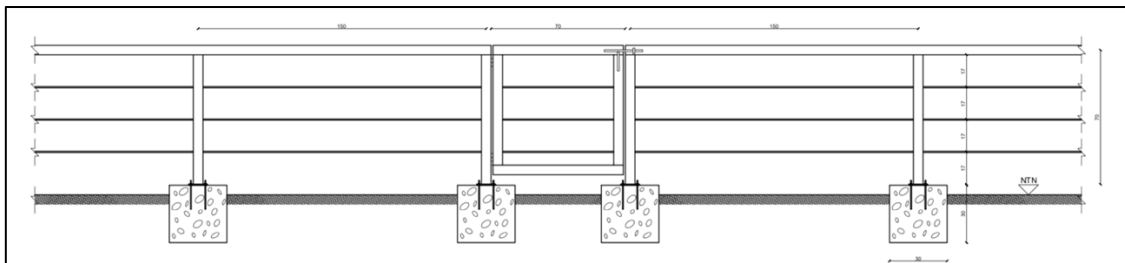
Imagen 12: Diseño propuesto cierres perimetrales de tumbas
