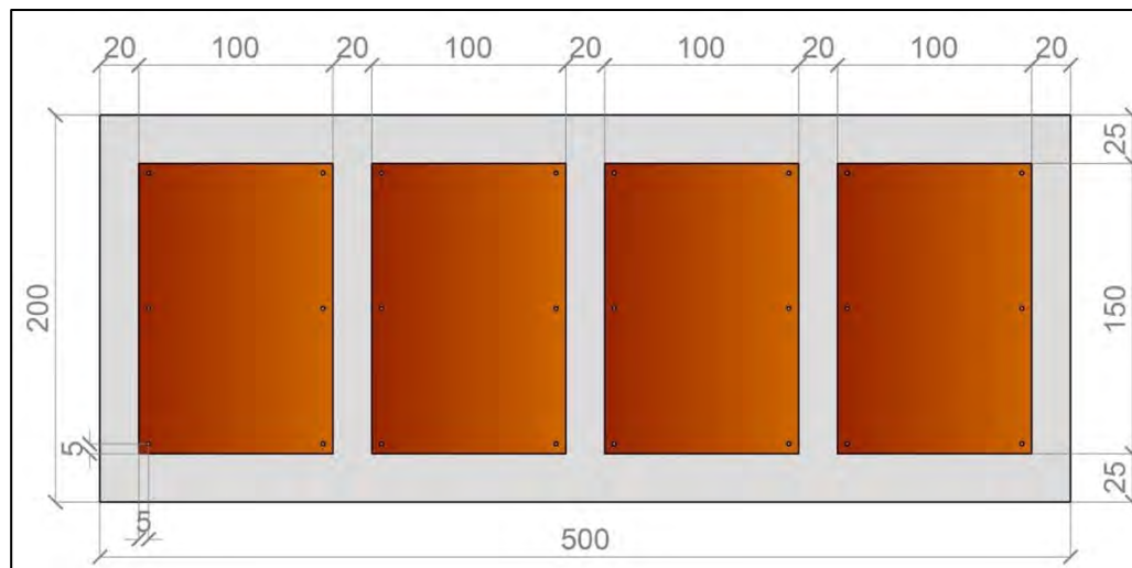
Imagen 7: Diseño propuesto de muro con 4 placas metálicas de 100 x 150 cm cada una
